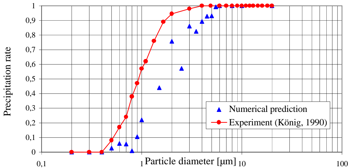
Trenngrad für den Z10 Zyklon, u_{F,in} = 10 \text{ m/s}
