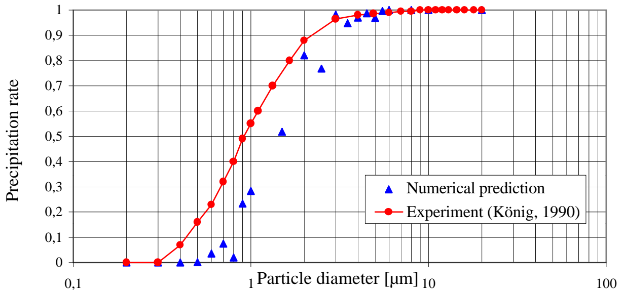
Trenngrad für den Z20 Zyklon, u_{F,in} = 10 \text{ m/s}
