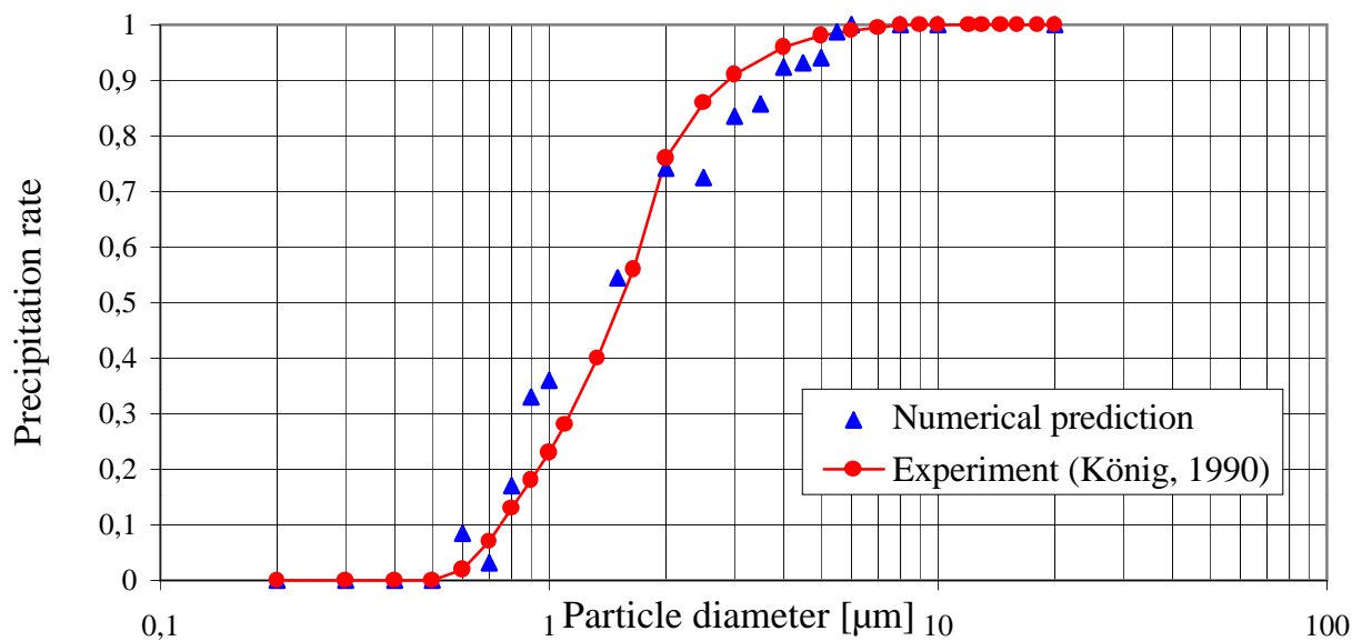
Trenngrad für den Z80 Zyklon, u_{F,in} = 10 \text{ m/s}
