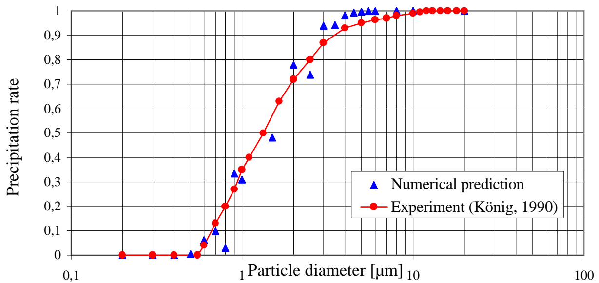
Trenngrad für den Z40 Zyklon, u_{F,in} = 10 \text{ m/s}
